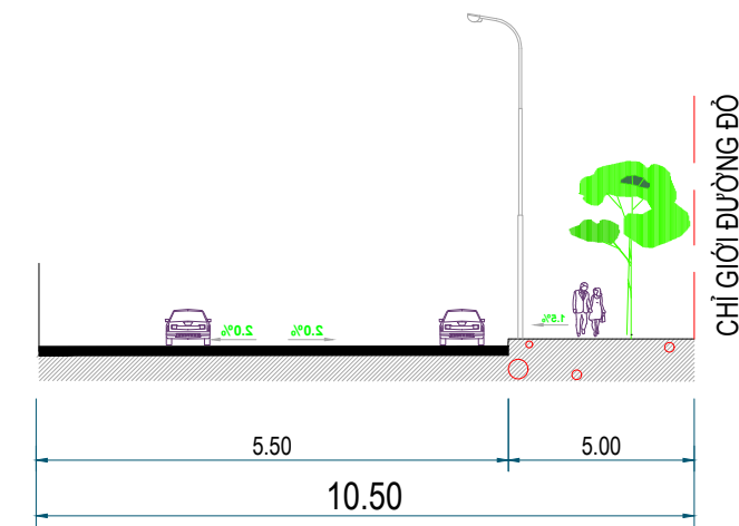
MẶT CẮT 3 - 3
