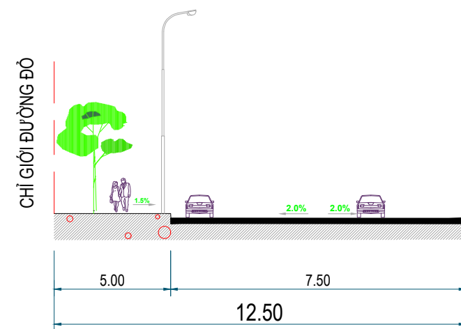
MẶT CẮT 4 - 4
