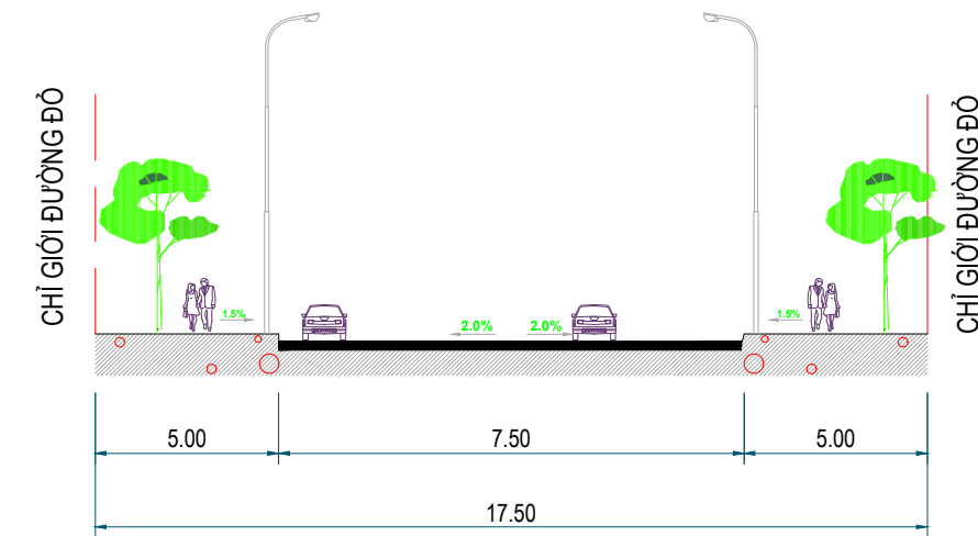
MẶT CẮT 1 - 1
