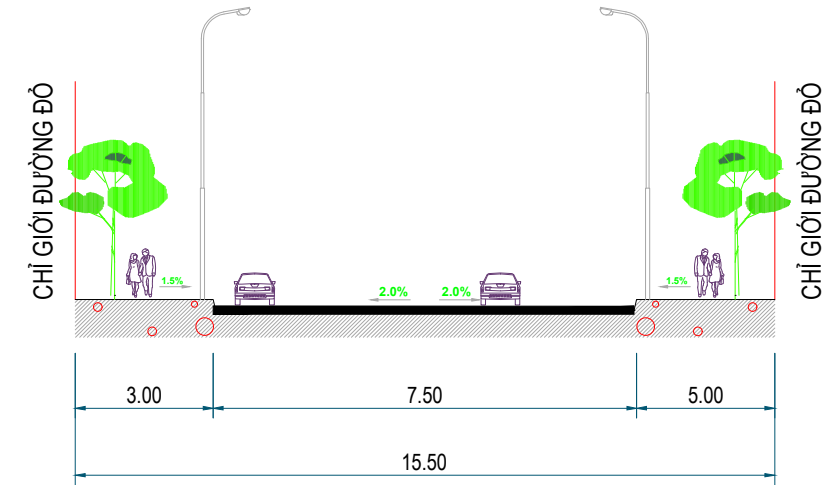
MẶT CẮT 2 - 2
